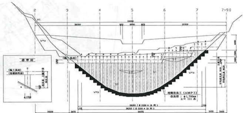
縦断面図
